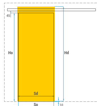
Az ajtólap csatlakozása az alumínium sínhez
