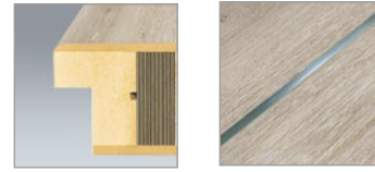
falcolt lekerekített „PF” ajtólap élkialakítás CPL
